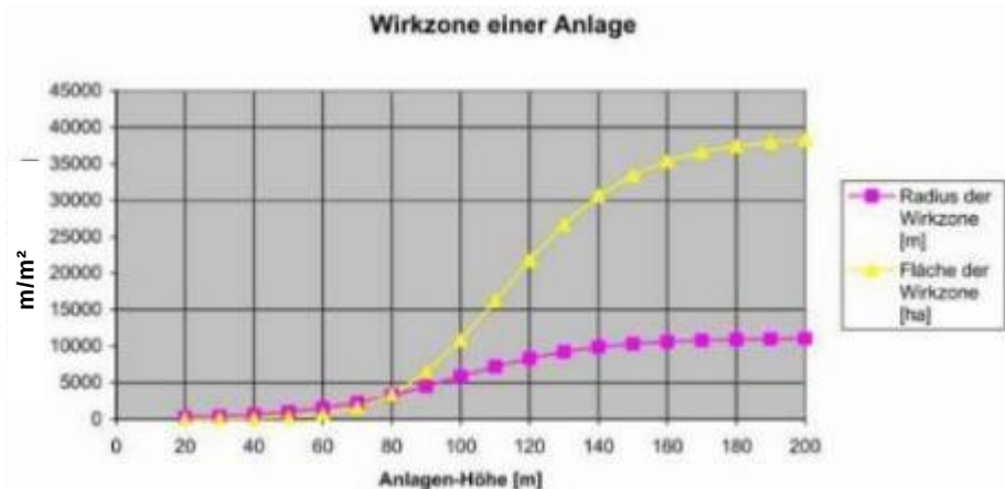
Abb. 5: Radius und Fläche der Wirkzone einer WEA in Abhängigkeit der Anlagenhöhe (DNR 2012)
