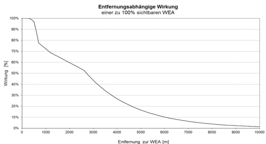
Abb. 6: Bewertungsgraph des Wirkzusammenhangs zwischen Entfernung und Wahrnehmungsstärke (Brahms & Peters 2012)
