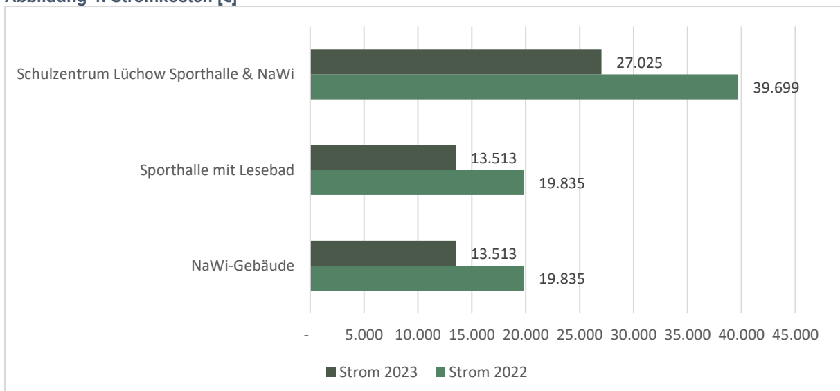
Abbildung 4: Stromkosten [€]
